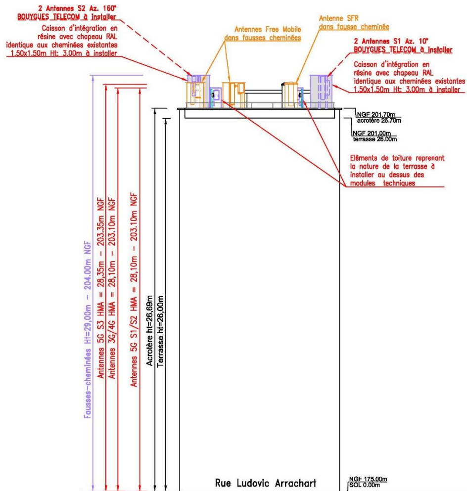
PLAN EN ELEVATION DE L'INSTALLATION BOUYGUES TELECOM
