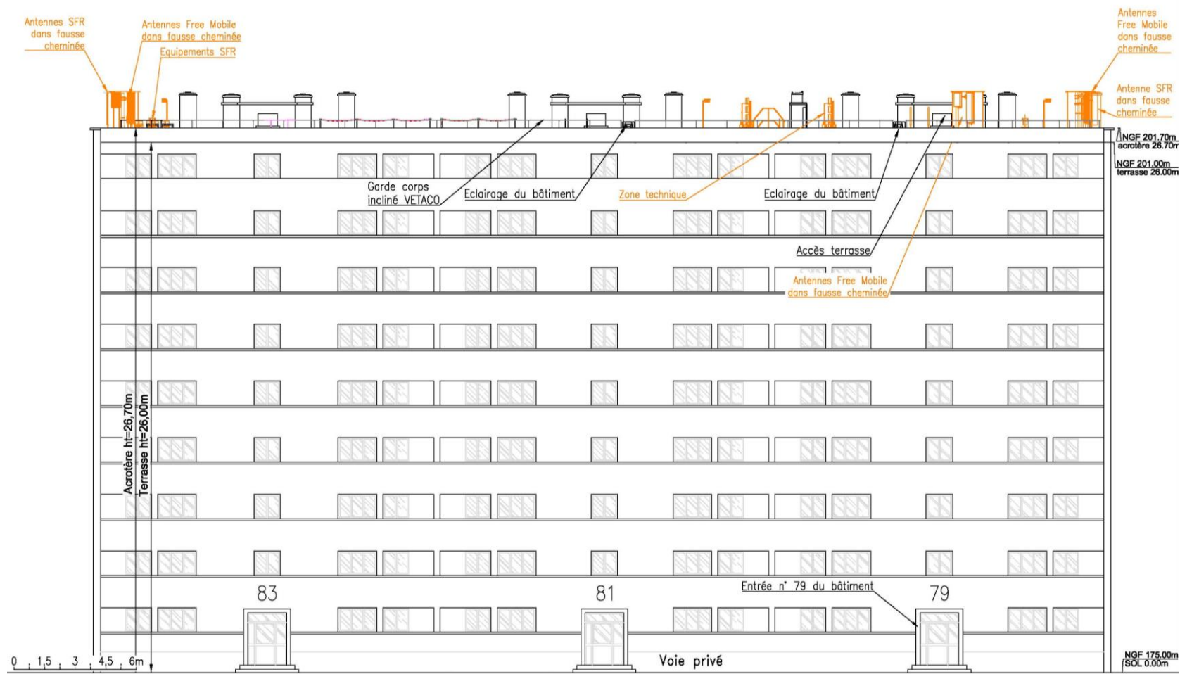
PLAN EN ELEVATION DES INSTALLATIONS EXISTANTES
