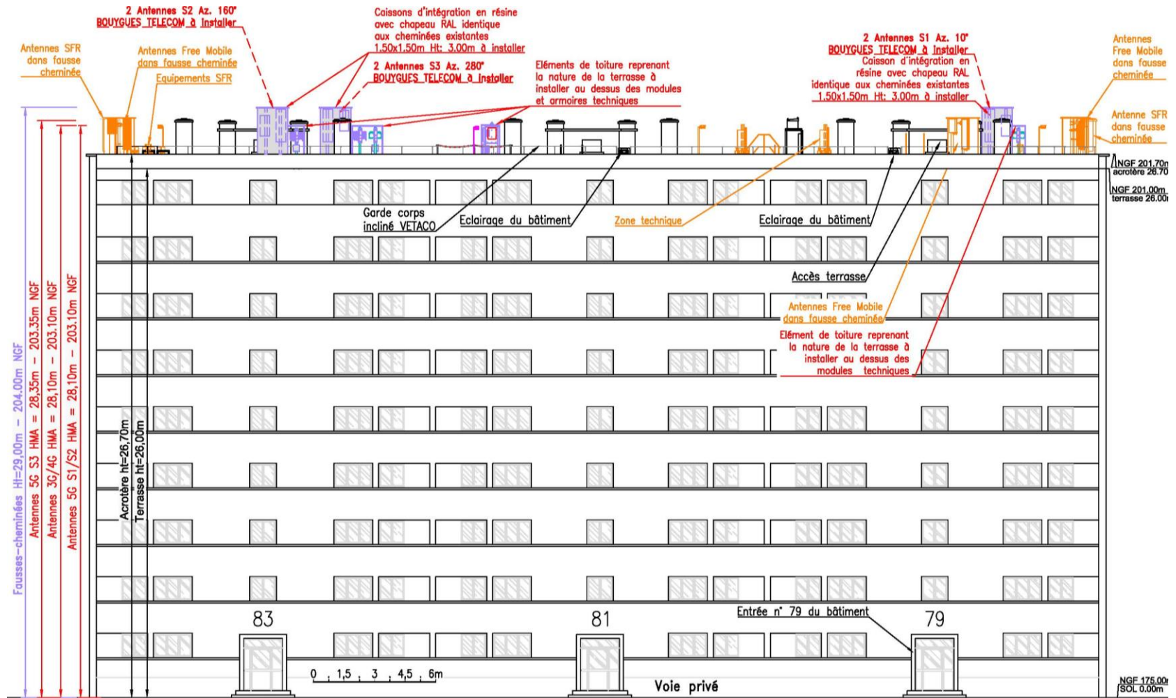
PLAN EN ELEVATION DE L'INSTALLATION BOUYGUES TELECOM
