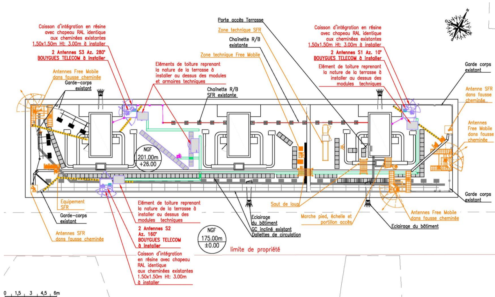
PLAN DE L'INSTALLATION BOUYGUES TELECOM
