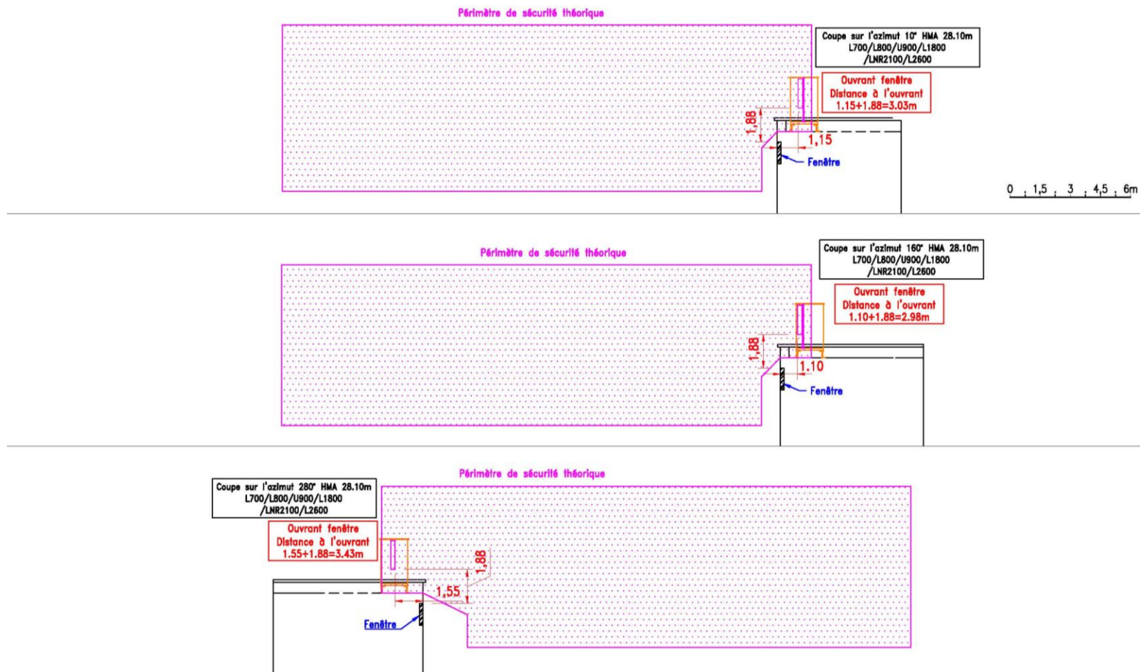
ILLUSTRATIONS DES DISTANCES ENTRE LES ANTENNES ET LES OUVERTURES DE L'IMMEUBLE
