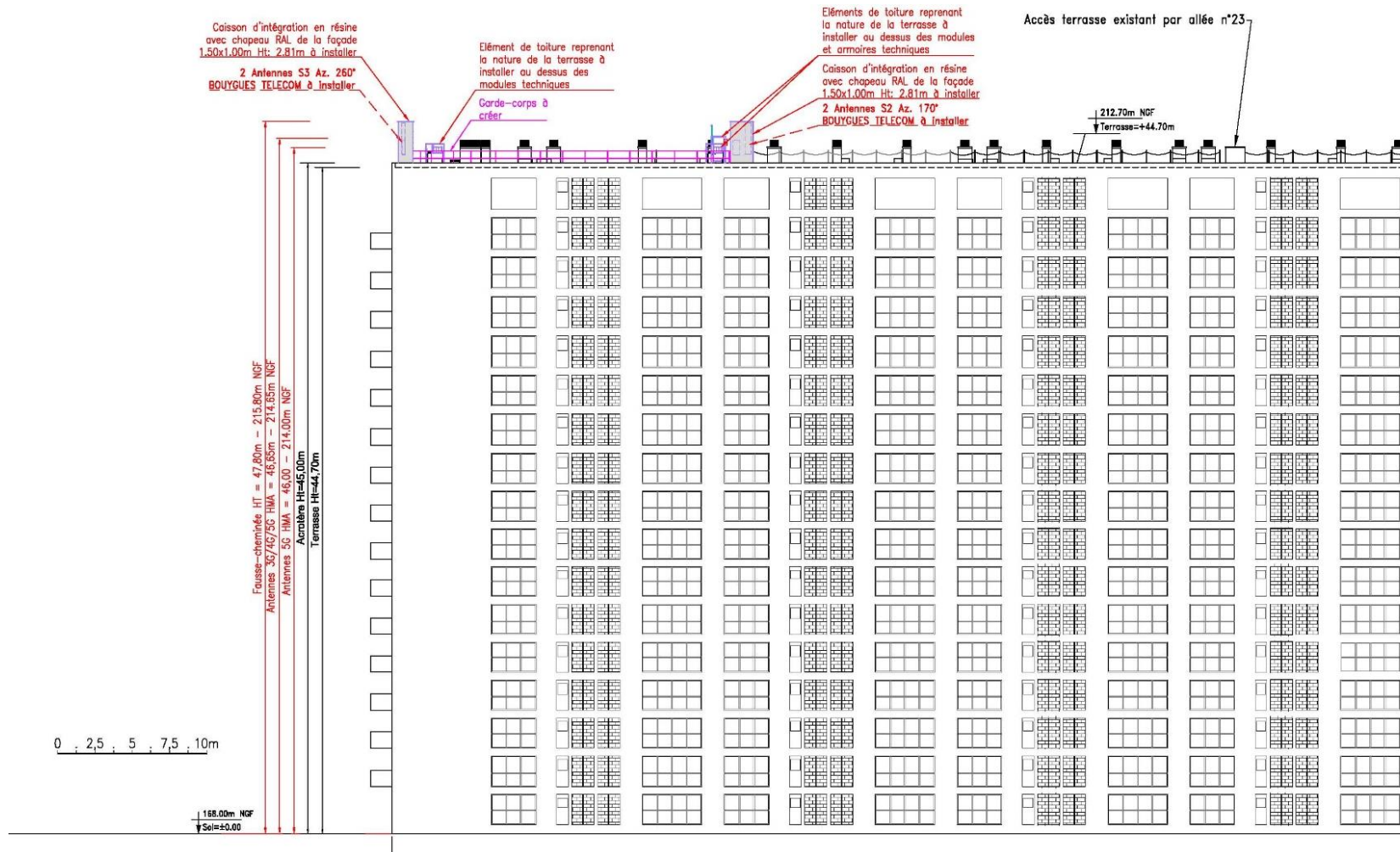
PLAN EN ELEVATION DE L'INSTALLATION BOUYGUES TELECOM
