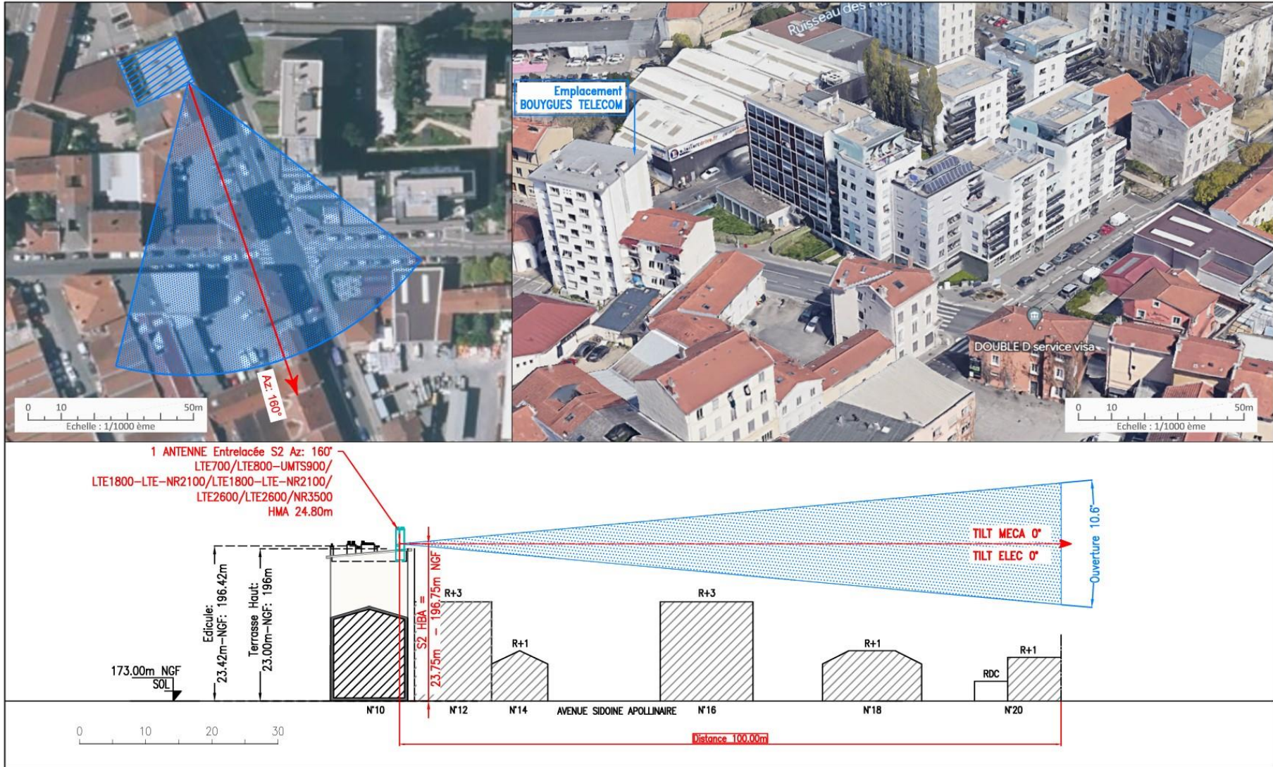
VUE EN COUPE DE L'AZIMUT 160°
