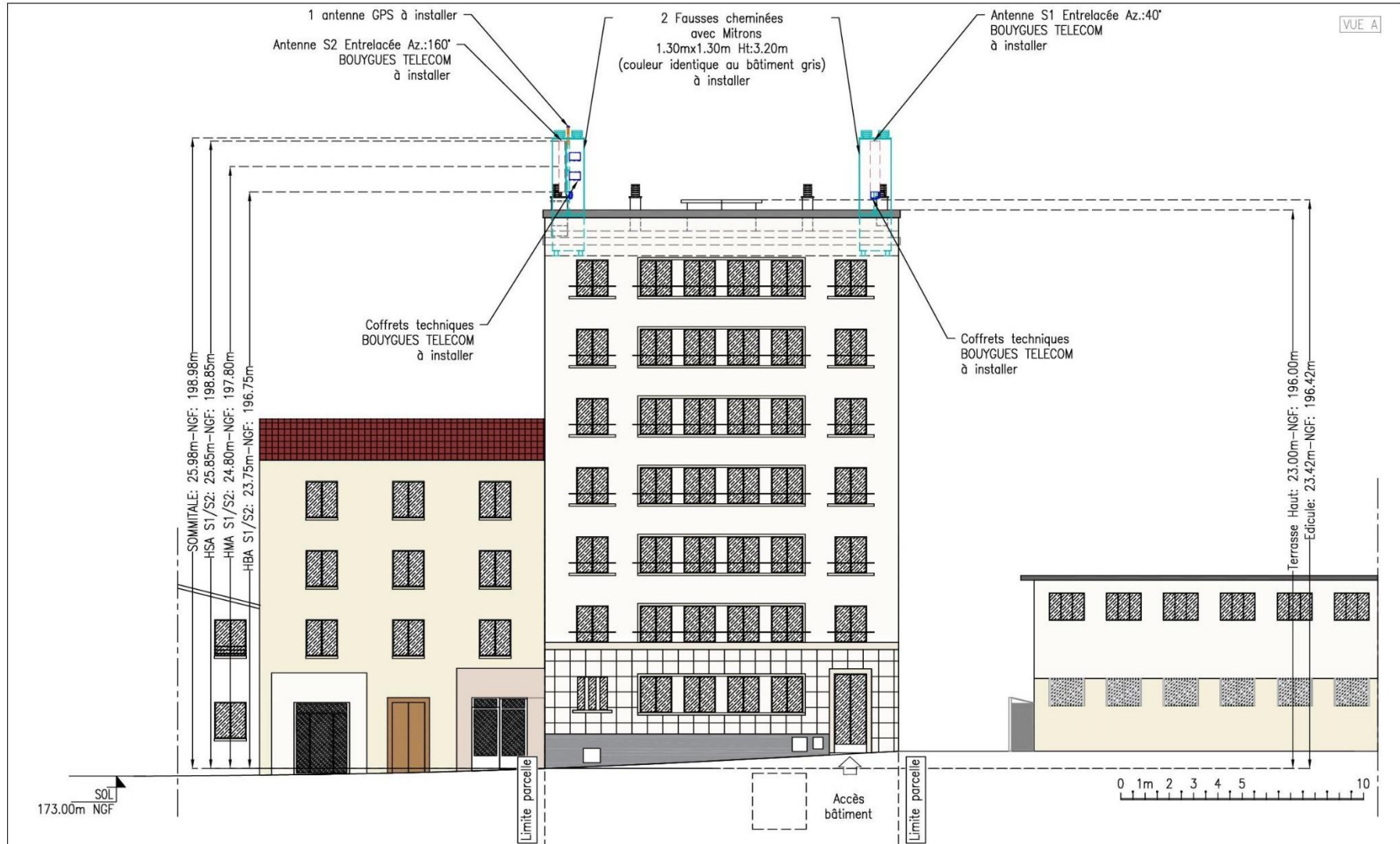
PLAN EN ELEVATION DES INSTALLATIONS PROJETES VUE A
