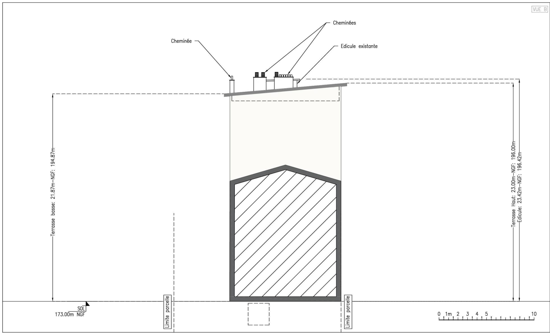
PLAN EN ELEVATION DES INSTALLATIONS EXISTANTES VUE B
