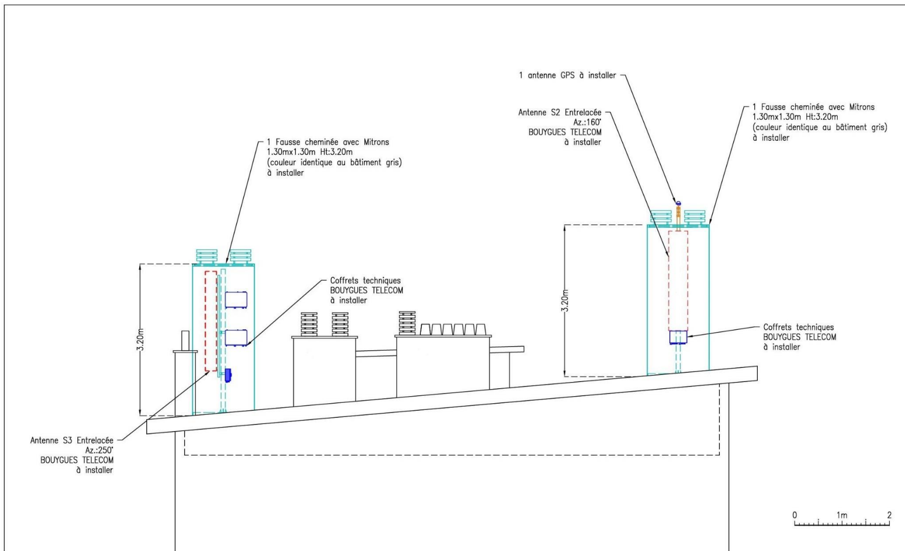
PLAN EN ELEVATION DETAILS DES FAUSSES CHEMINEES
