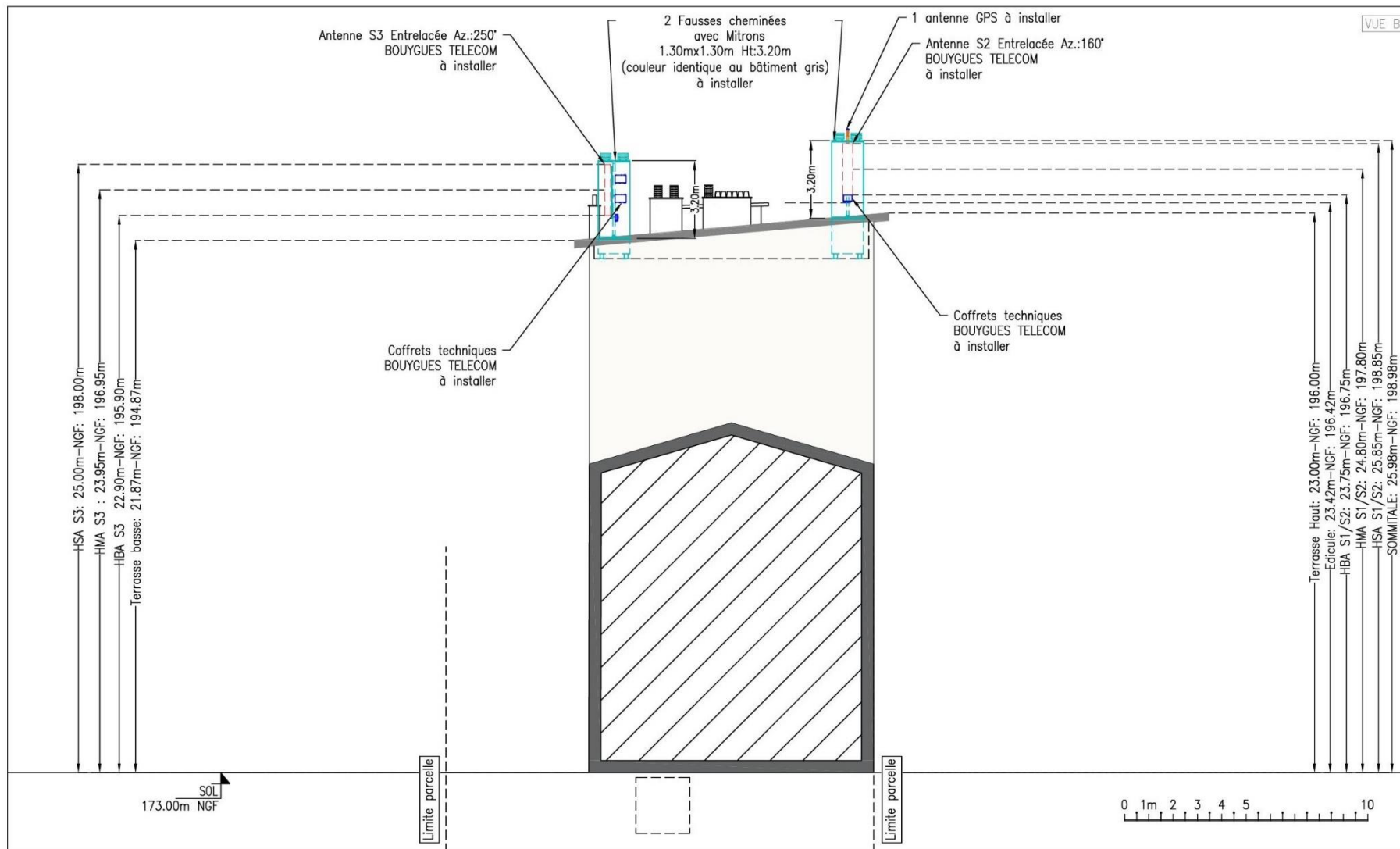
PLAN EN ELEVATION DES INSTALLATIONS PROJETES VUE B
