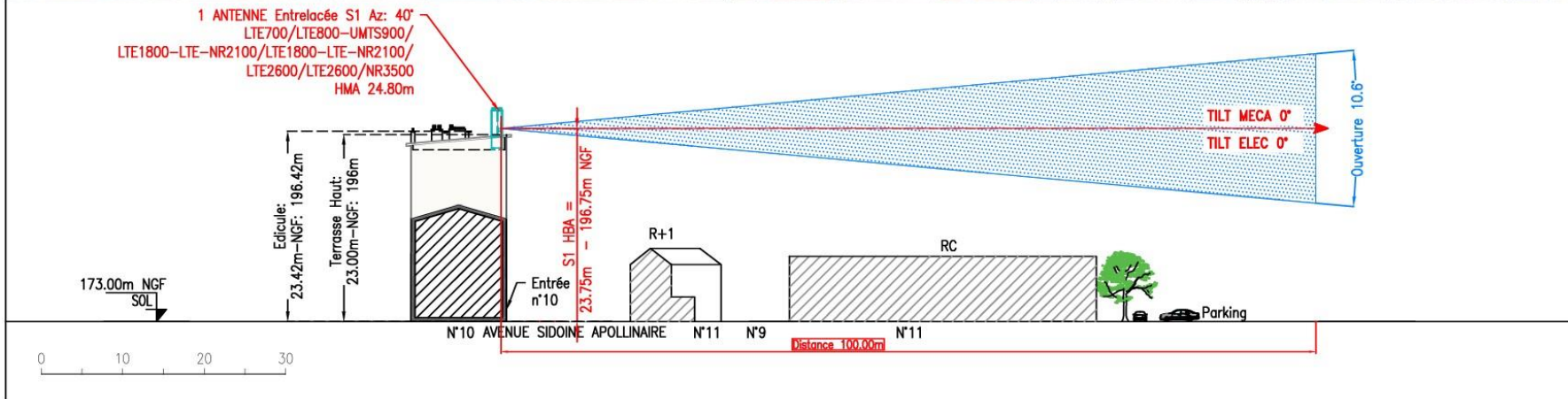
VUE EN COUPE DE L'AZIMUT 40°
