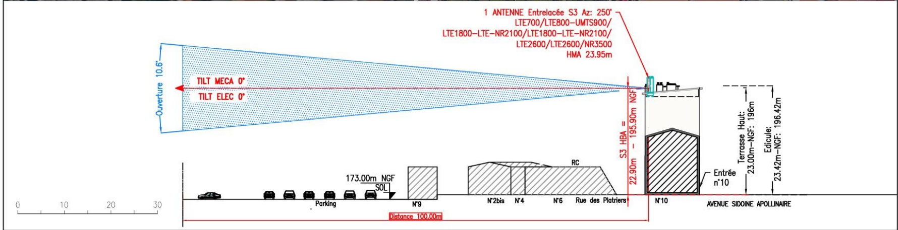
VUE EN COUPE DE L'AZIMUT 250°
