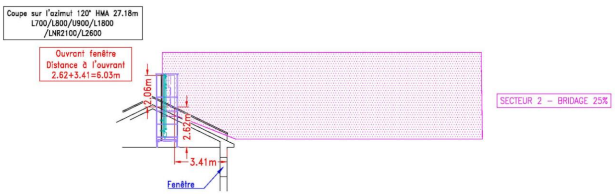
ILLUSTRATIONS DES DISTANCES ENTRE LES ANTENNES ET LES OUVERTURES DE L'IMMEUBLE
