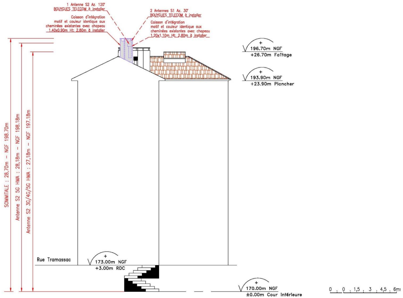
PLAN EN ELEVATION DE L'INSTALLATION BOUYGUES TELECOM
