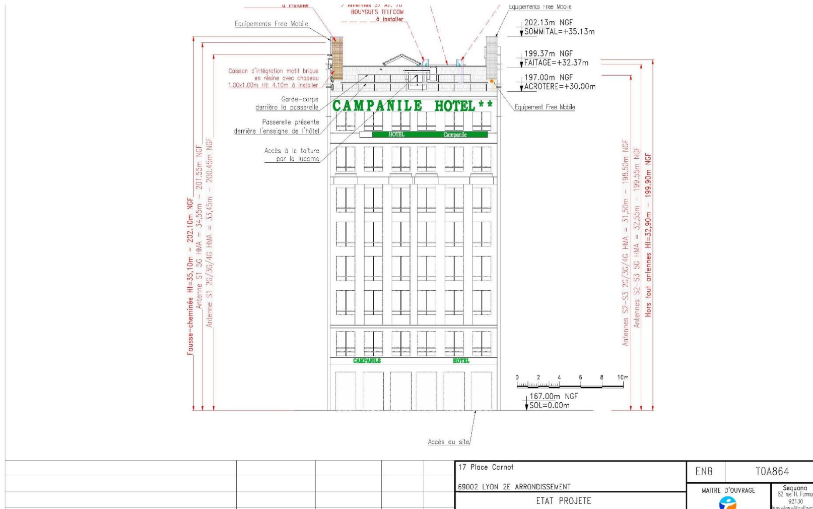
PLAN EN ELEVATION DE L'INSTALLATION BOUYGUES TELECOM
