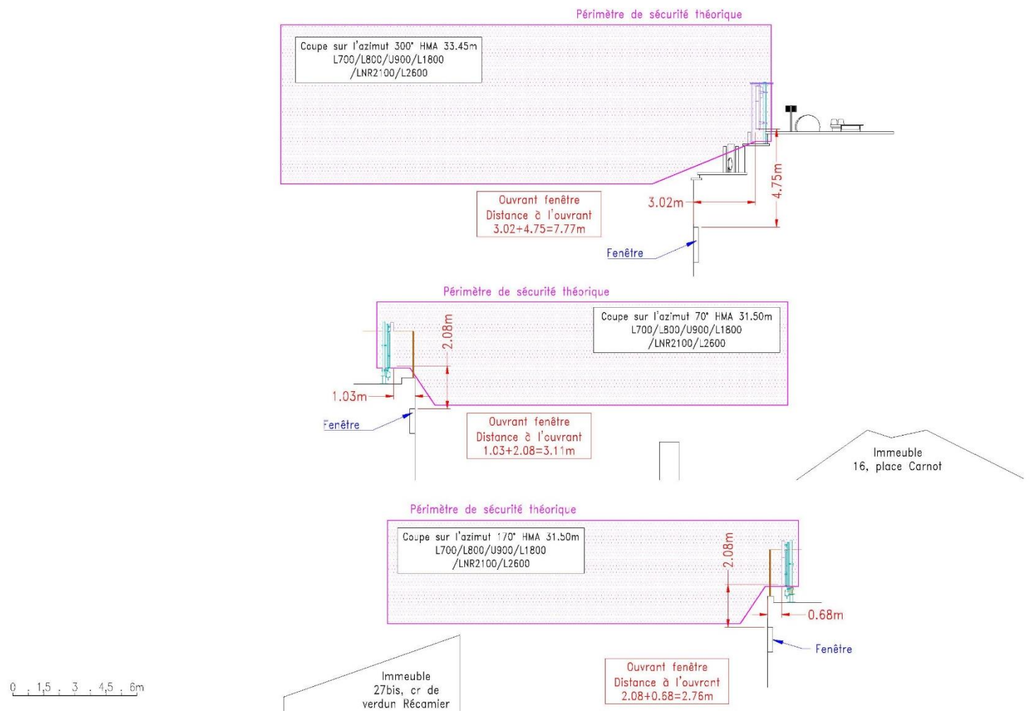
ILLUSTRATIONS DES DISTANCES ENTRE LES ANTENNES ET LES OUVERTURES DE L'IMMEUBLE
