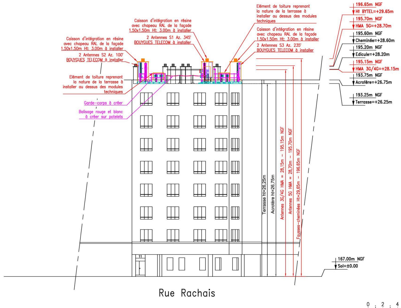
PLAN EN ELEVATION DE L'INSTALLATION BOUYGUES TELECOM
