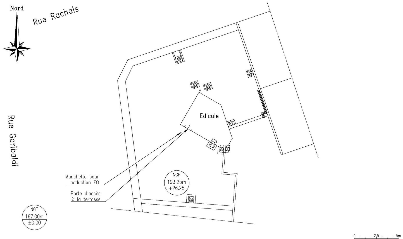
PLAN DES INSTALLATIONS EXISTANTES
