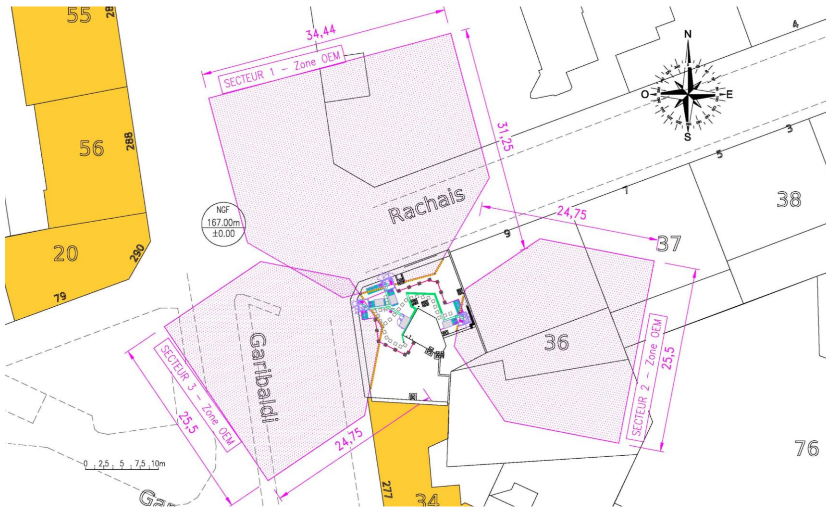
PLAN DES PERIMETRES DE SECURITE
