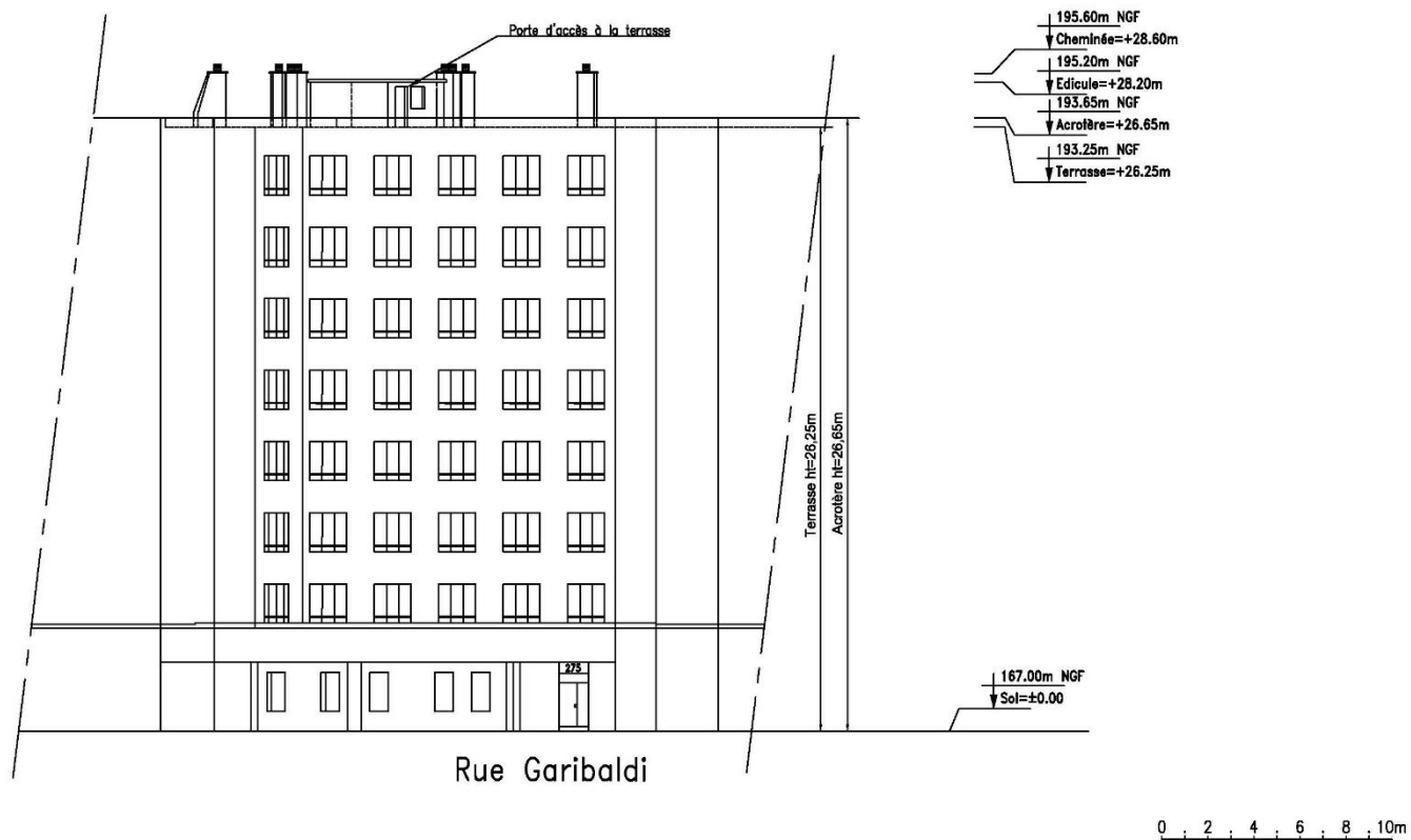
PLAN EN ELEVATION DES INSTALLATIONS EXISTANTES
